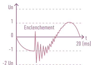
Onde typique de surtension de manœuvre
